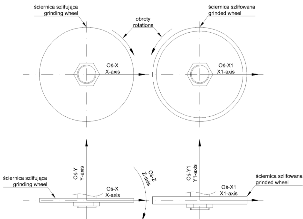
Rysunek 1. Schemat szlifowania
